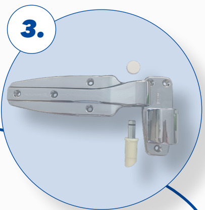
Plastikdeckel und Steigeinsatz herausziehen / lösen
